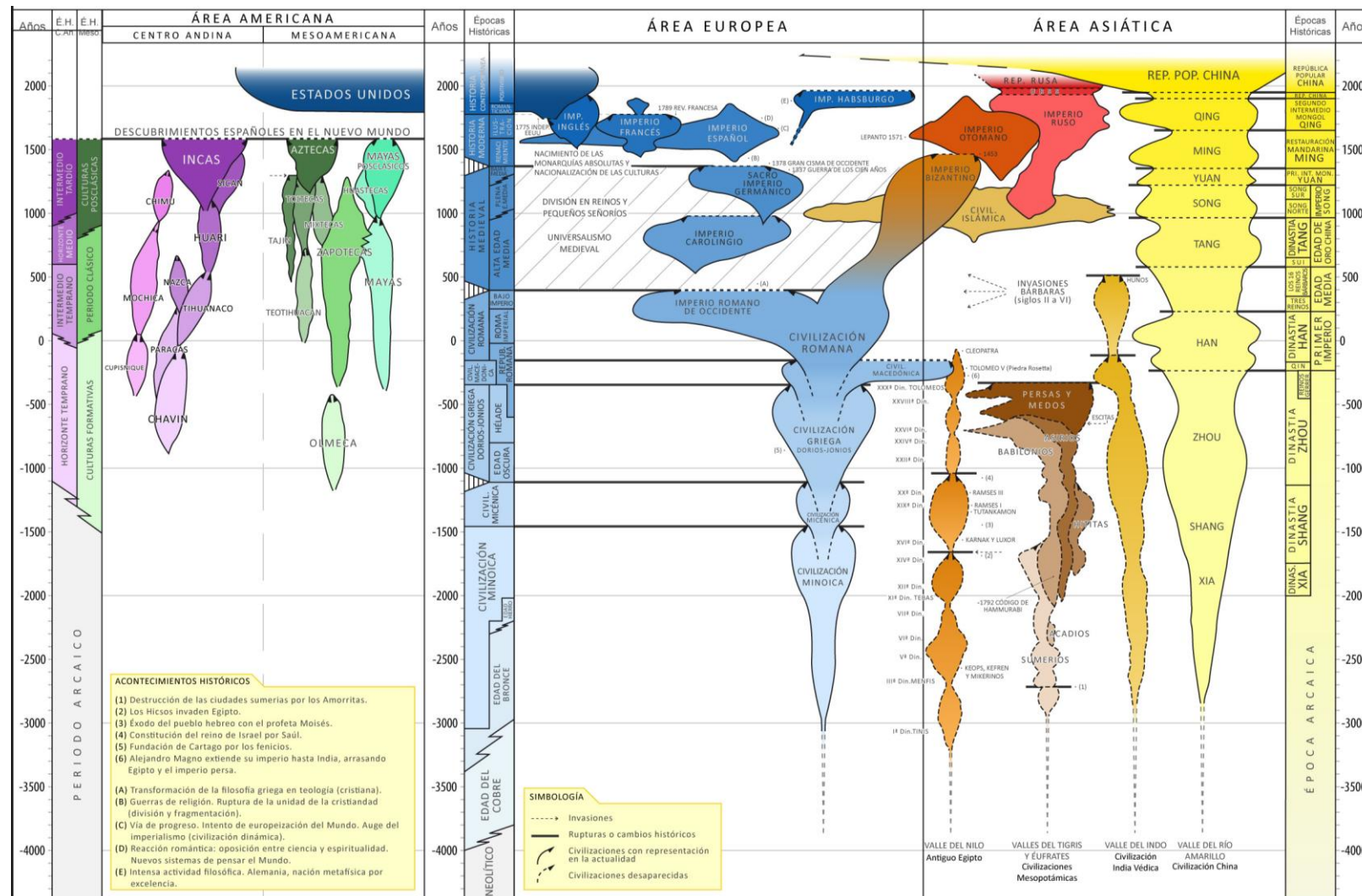
Figura 1. Esquema evolutivo de las principales civilizaciones.
