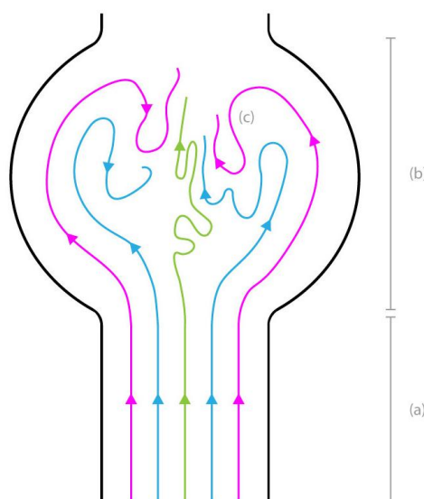
Figura 3. Estructuras deformativas. a. Corriente laminar. b. Movimiento turbillónar. c. Bucles reaccionarios.
