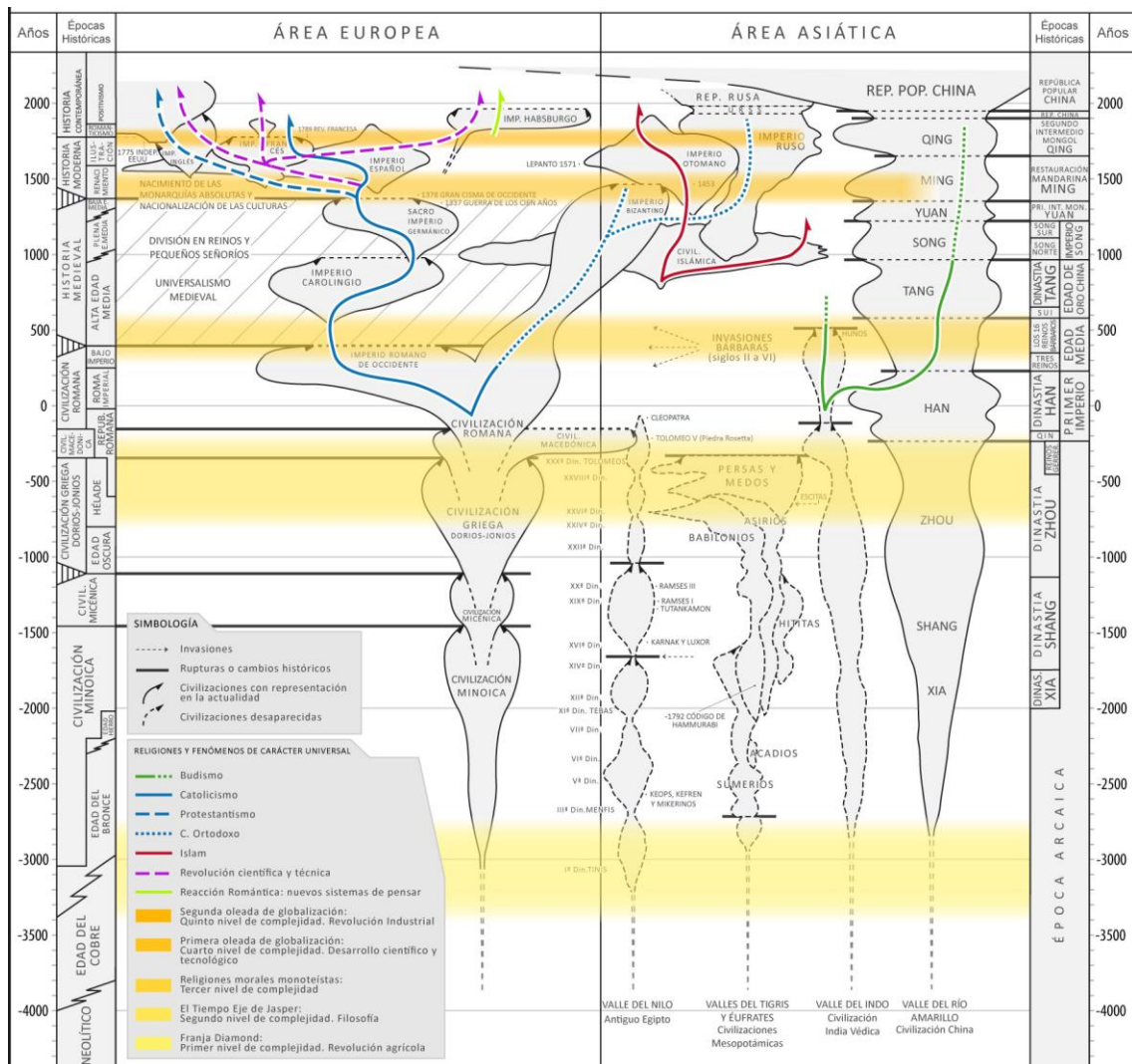
Figura 2. Fenómenos de carácter universal en el desarrollo de las civilizaciones.
